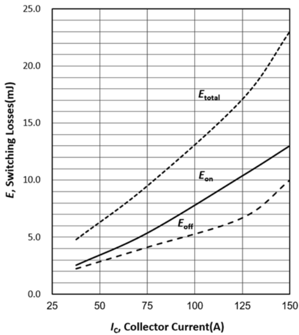
图 5 开关损耗与集电极电流的关系 (感性负载, T_{vj}=25^{\circ}\text{C} , V_{CE}=600\text{V} , V_{GE}=0/15\text{V} , R_G=7.5\ \Omega )
