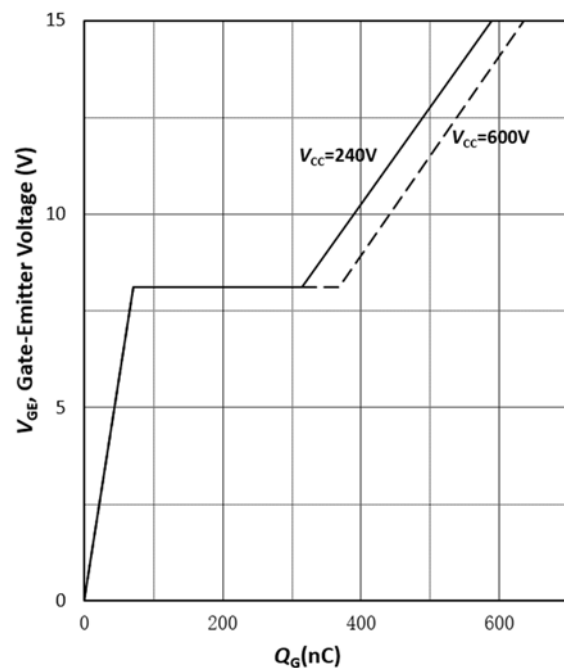
图 8 栅电荷特性
