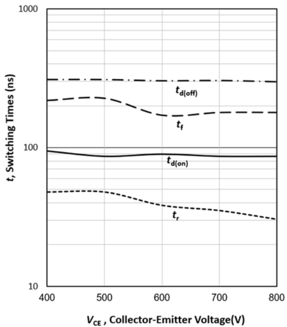
图 4 开关时间与集电极-发射极电压的关系 (感性负载, T_{vj}=25^{\circ}\text{C} , V_{GE}=0/15\text{V} , I_C=75\text{A} , R_G=7.5\ \Omega )
