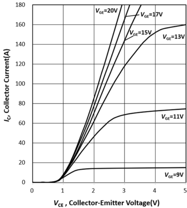
图 1 IGBT 输出特性 ( T_{vj}=25^{\circ}\text{C} )
