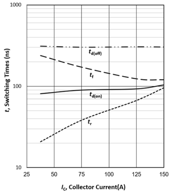
图 2 开关时间与集电极电流的关系 (感性负载, T_{vj}=25^{\circ}\text{C} , V_{CE}=600\text{V} , V_{GE}=0/15\text{V} , R_G=7.5\ \Omega )
