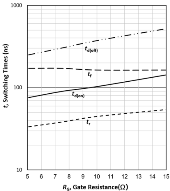
图 3 开关时间与栅极电阻的关系 (感性负载, T_{vj}=25^{\circ}\text{C} , V_{CE}=600\text{V} , V_{GE}=0/15\text{V} , I_C=75\text{A} )
