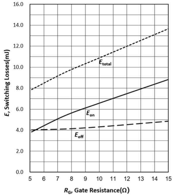
图 6 开关损耗与栅极电阻的关系 (感性负载, T_{vj}=25^{\circ}\text{C} , V_{CE}=600\text{V} , V_{GE}=0/15\text{V} , I_C=75\text{A} )
