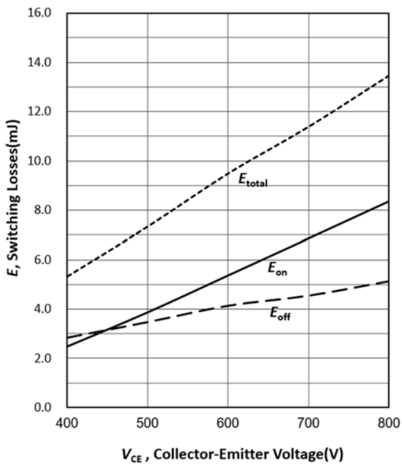
图 7 开关损耗与集电极-发射极电压的关系 (感性负载, T_{vj}=25^{\circ}\text{C} , V_{GE}=0/15\text{V} , I_C=75\text{A} , R_G=7.5\ \Omega )
