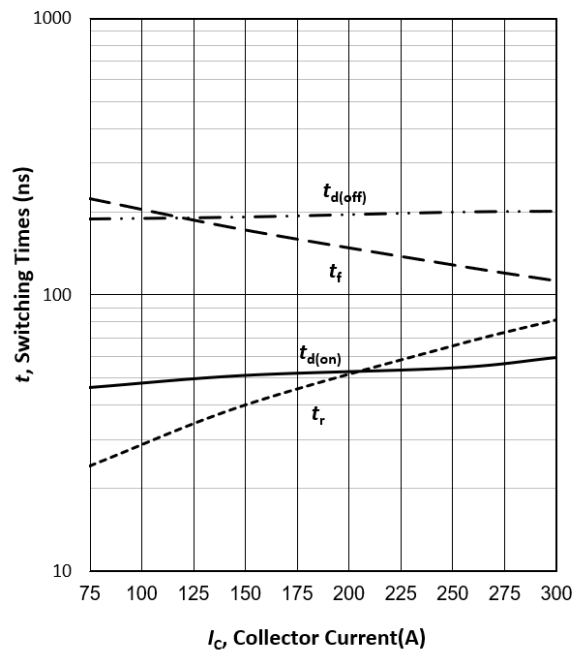
图 2 IGBT 开关时间与集电极电流的关系 (感性负载, T_j=25^{\circ}\text{C} , V_{CE}=600\text{V} , V_{GE}=-15/15\text{V} , R_G=5.1\ \Omega )
