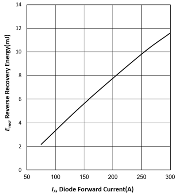
图 6 二极管反向恢复损耗与正向电流的关系 ( T_{vj}=25^{\circ}\text{C} , V_{CE}=600\text{V} , R_G=5.1\ \Omega )
