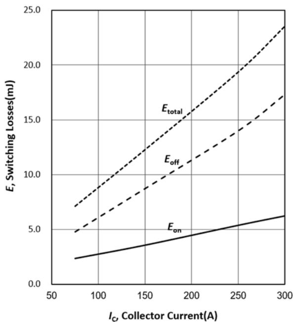
图 3 IGBT 开关损耗与集电极电流的关系 (感性负载, T_{vj}=25^{\circ}\text{C} , V_{CE}=600\text{V} , V_{GE}=-15/15\text{V} , R_G=5.1\ \Omega )
