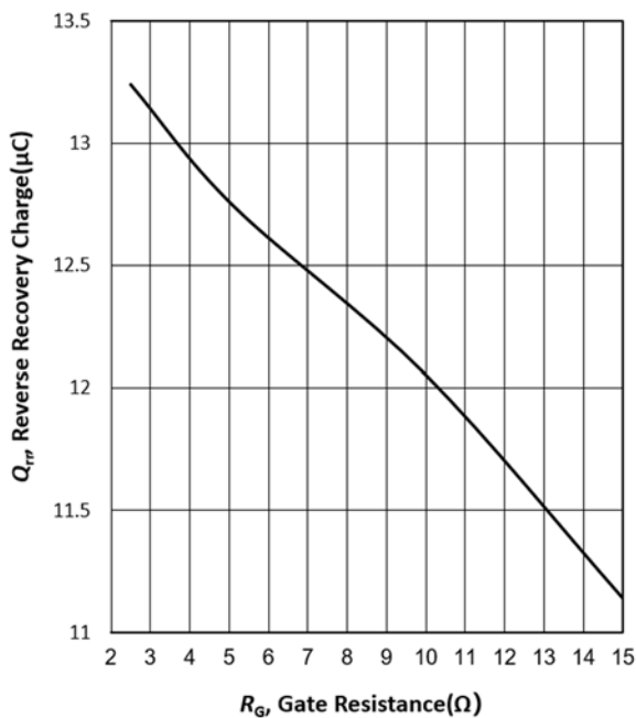
图 7 二极管反向恢复电荷与栅电阻的关系 ( T_{vj}=25^{\circ}\text{C} , V_{CE}=600\text{V} , I_F=150\text{A} )
