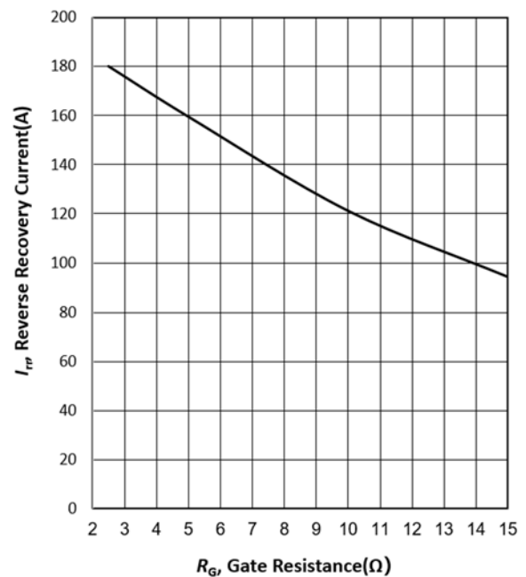
图 8 二极管反向恢复峰值电流与栅电阻的关系 ( T_{vj}=25^{\circ}\text{C} , V_{CE}=600\text{V} , I_F=150\text{A} )
