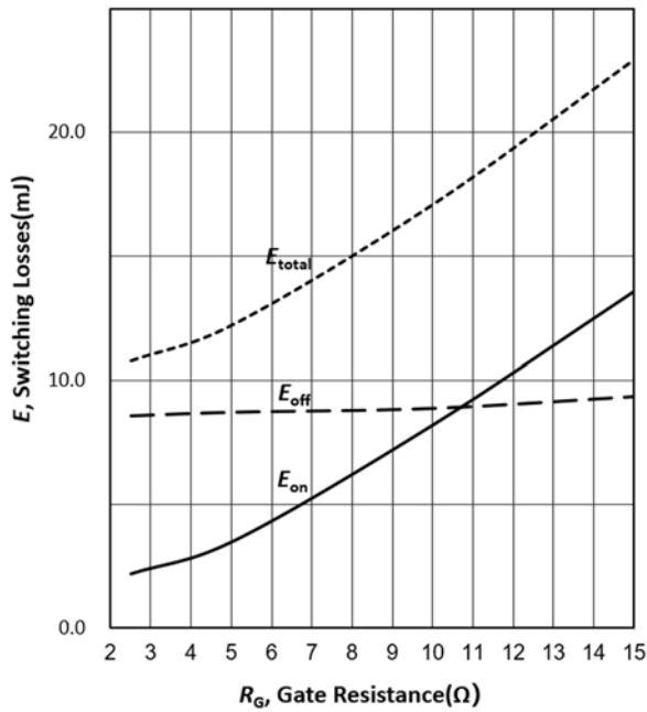
图 5 IGBT 开关损耗与栅极电阻的关系 (感性负载, T_{vj}=25^{\circ}\text{C} , V_{CE}=600\text{V} , V_{GE}=-15/15\text{V} , I_C=150\text{A} )
