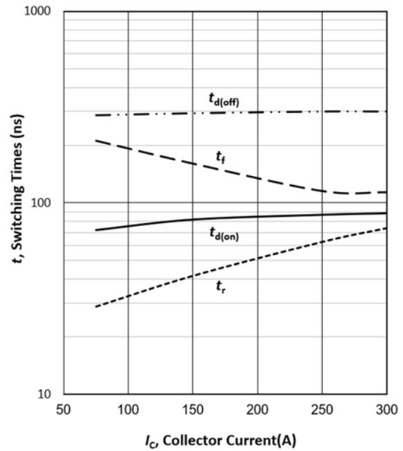
图 2 IGBT 开关时间与集电极电流的关系 (感性负载, T_{vj}=25^{\circ}\text{C} , V_{CE}=600\text{V} , V_{GE}=-15/15\text{V} , R_G=5.1\ \Omega )
