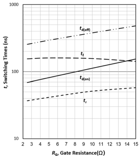
图 4 IGBT 开关时间与栅极电阻的关系 (感性负载, T_{vj}=25^{\circ}\text{C} , V_{CE}=600\text{V} , V_{GE}=-15/15\text{V} , I_C=150\text{A} )
