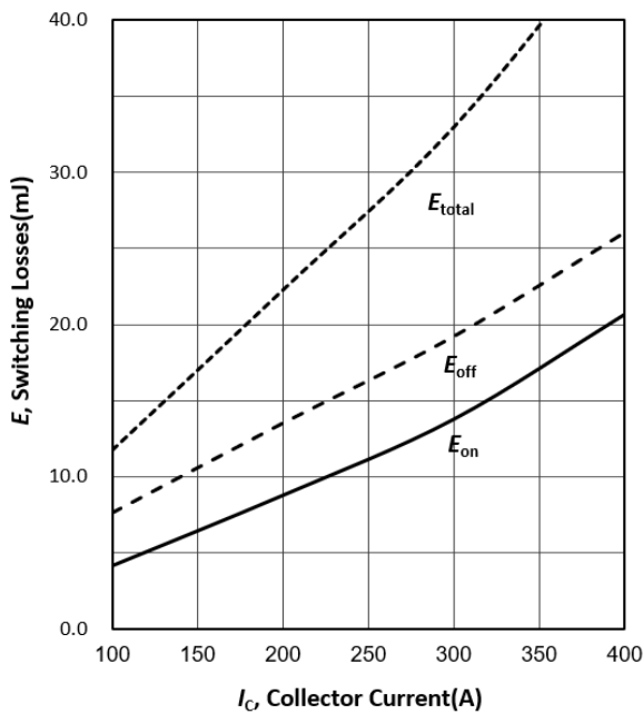
图 3 IGBT 开关损耗与集电极电流的关系 (感性负载, T_j=25^{\circ}C , V_{CE}=600V, V_{GE}=-15/15V, R_G=2.5 \Omega )
