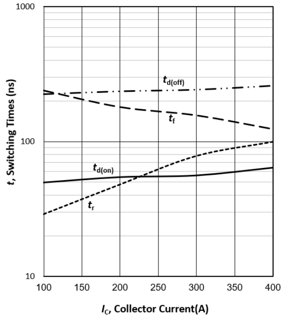
图 2 IGBT 开关时间与集电极电流的关系 (感性负载, T_j=25^{\circ}C , V_{CE}=600V, V_{GE}=-15/15V, R_G=2.5 \Omega )
