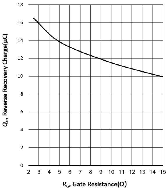
图 7 二极管反向恢复电荷与栅电阻的关系 ( T_j=25^\circ\text{C} , V_{CE}=600\text{V} , I_F=200\text{A} )
